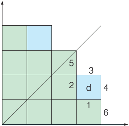
Domain D' = D + d
