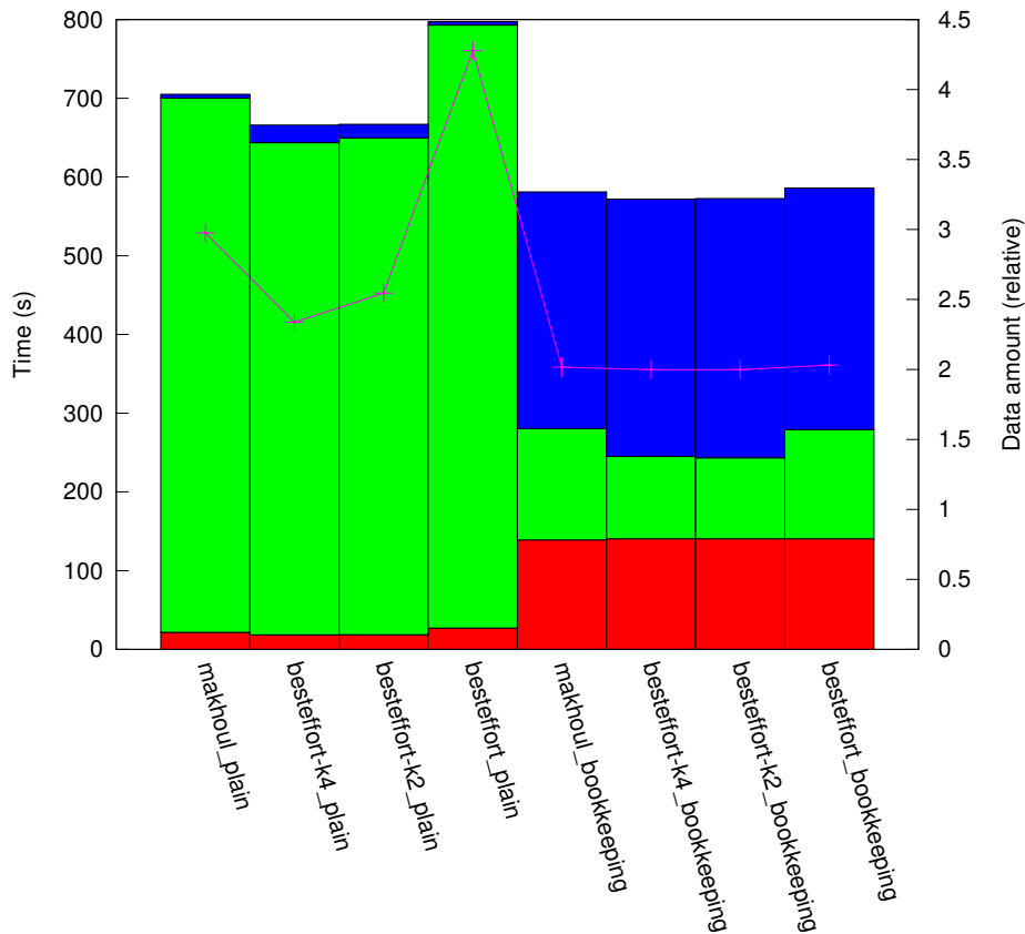
results_l1_1:10/plat_grid16/topo_torus
