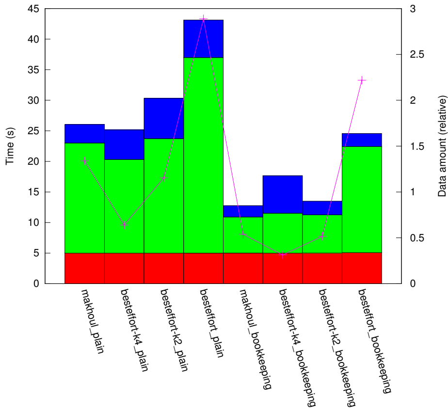
results_RN_10:1/plat_grid16/topo_torus
