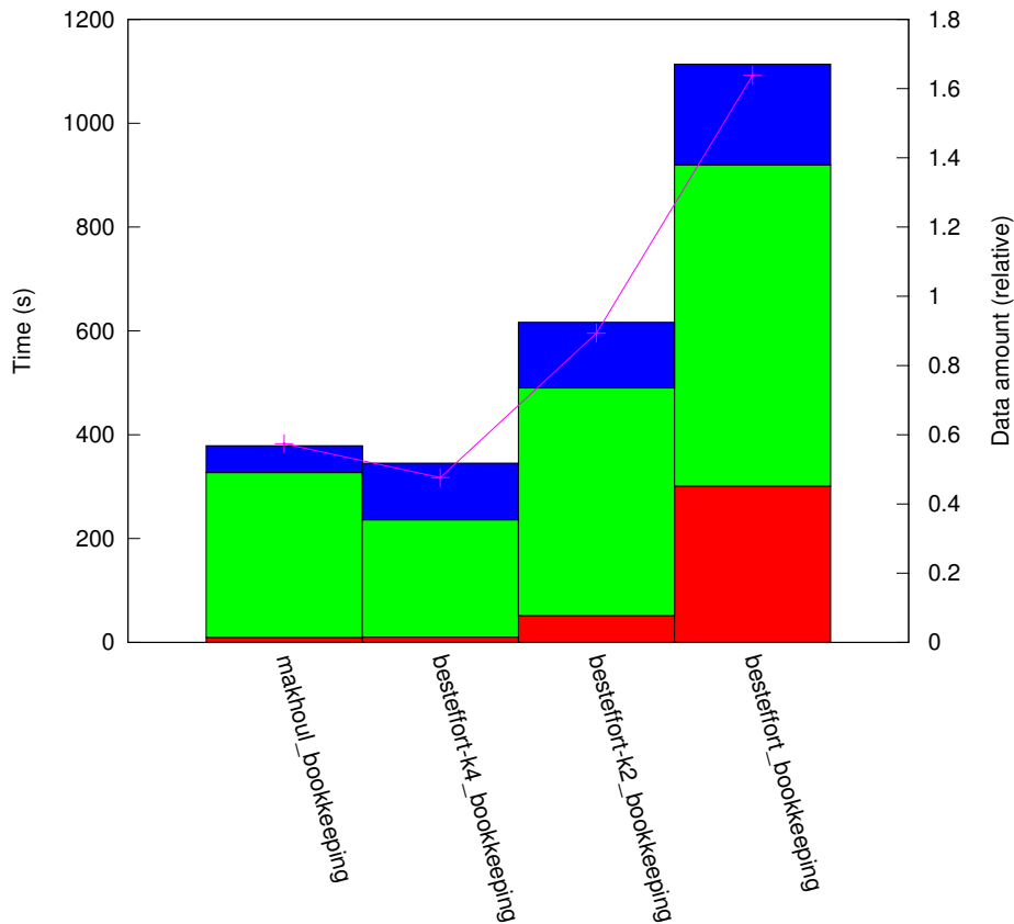
results_RN_1:10/plat_cluster1024/topo_hcube
