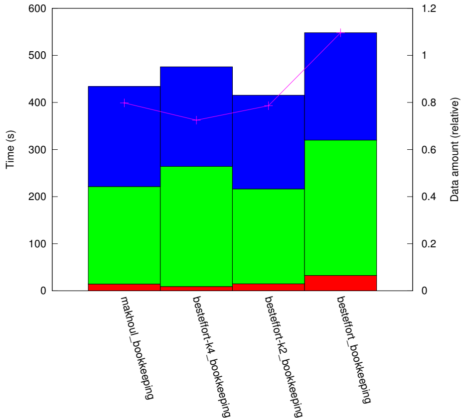
results_RN_1:10/plat_grid1024/topo_torus
