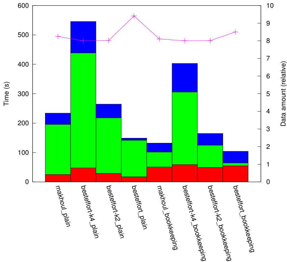
results_l1_10:1/plat_cluster256/topo_torus
