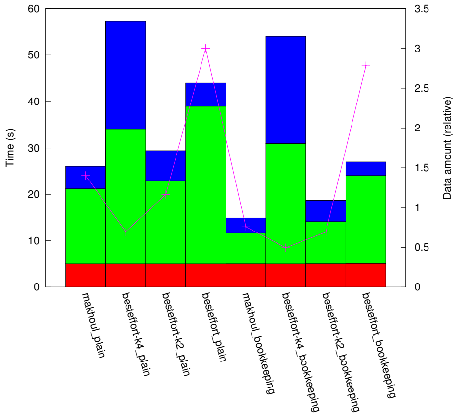
results_RN_10:1/plat_cluster64/topo_torus
