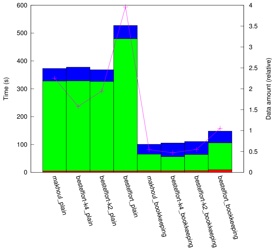
results_IN_1:10/plat_cluster64/topo_torus
