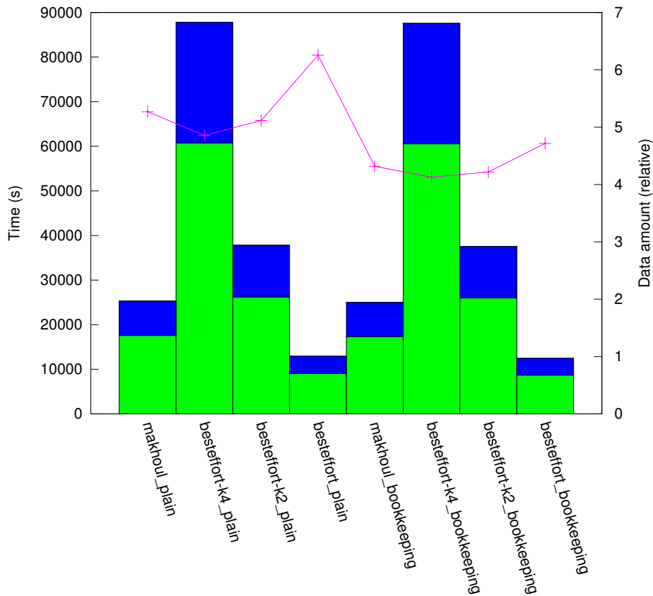
results_RN_1:10/plat_cluster256/topo_line
