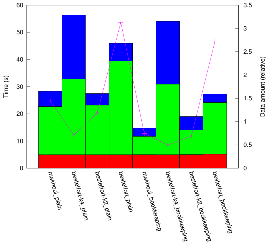
results_RN_10:1/plat_grid64/topo_torus
