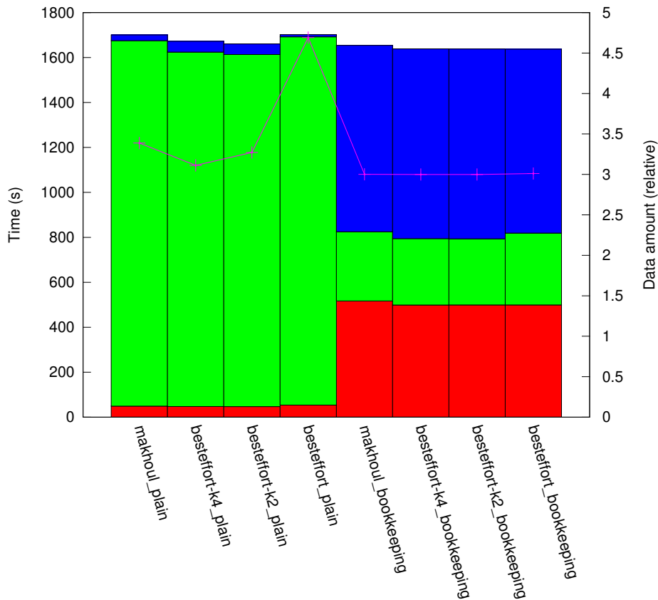
results_l1_1:10/plat_grid64/topo_hcube
