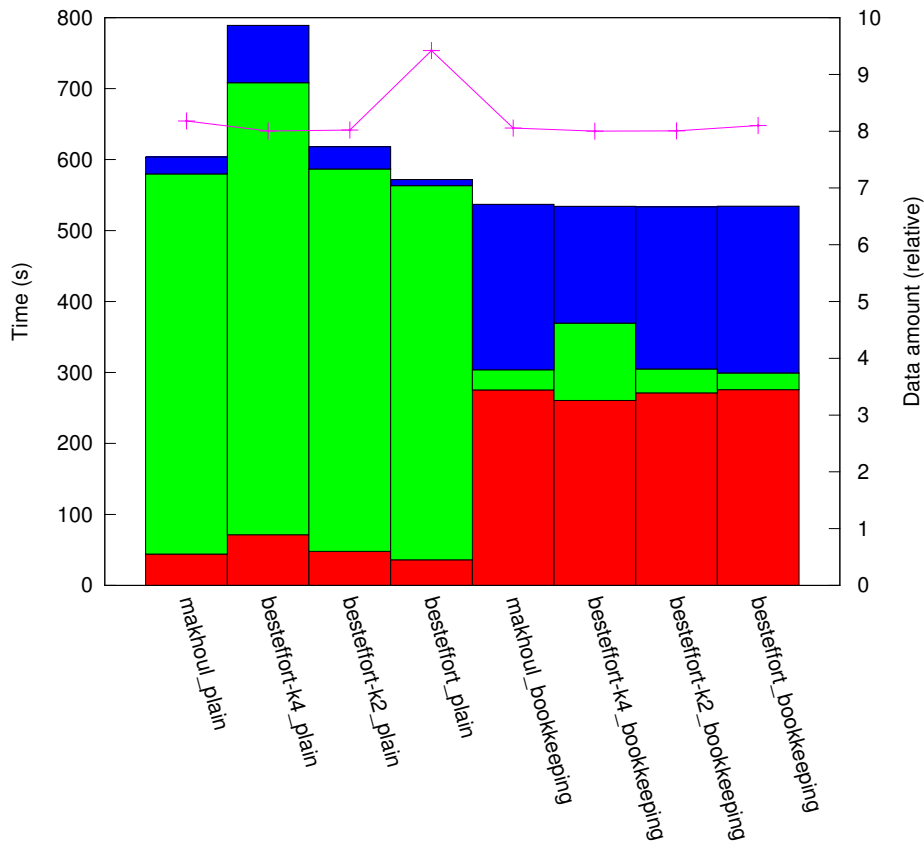
results_R1_1:1/plat_cluster256/topo_torus
