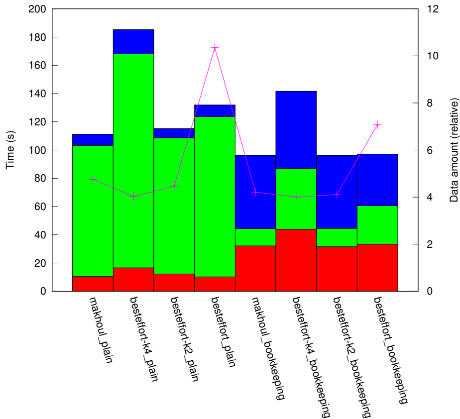
results_R1_10:1/plat_grid256/topo_hcube
