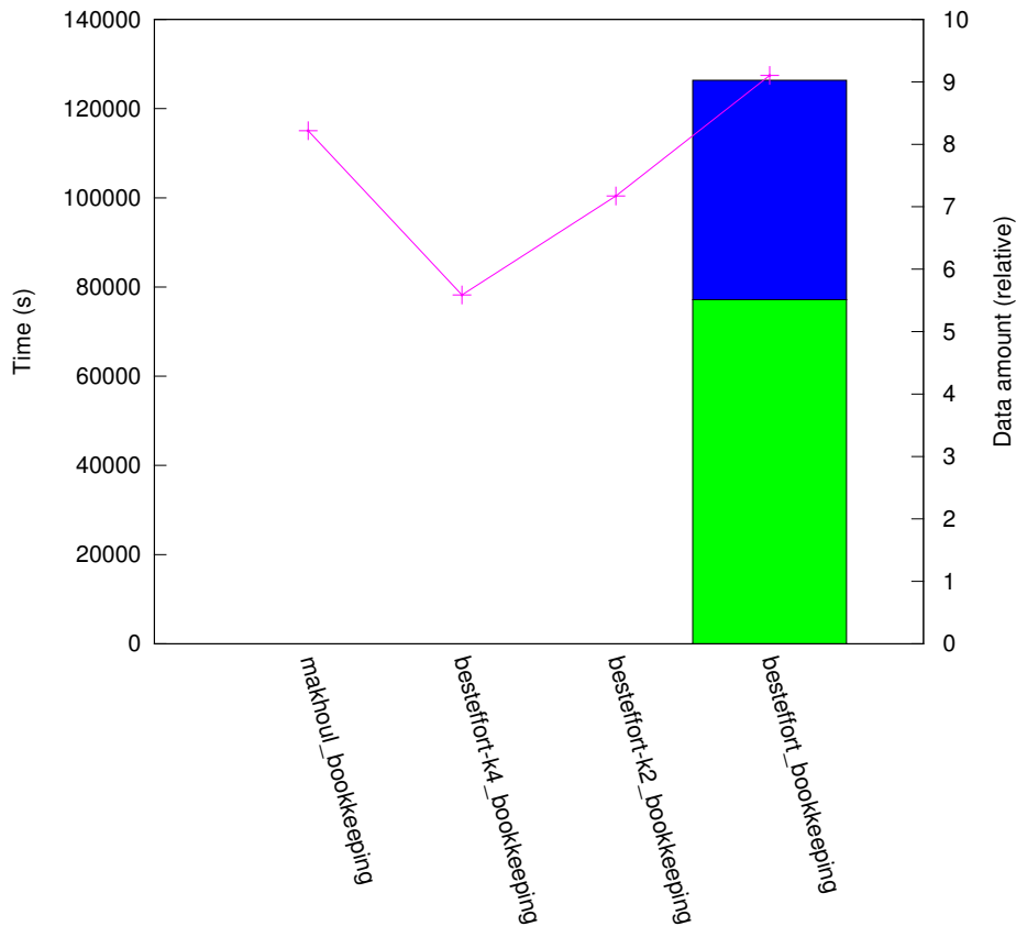
results_RN_10:1/plat_cluster1024/topo_line
