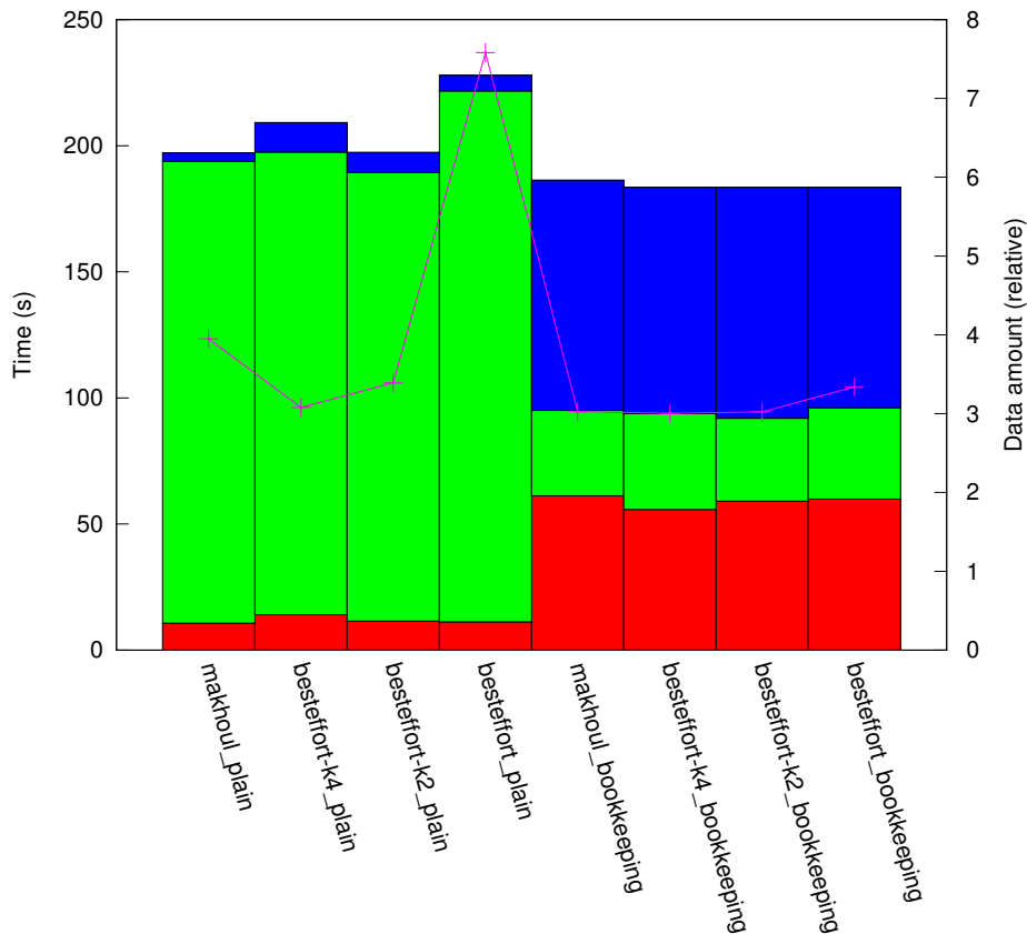
results_R1_1:1/plat_grid64/topo_hcube
