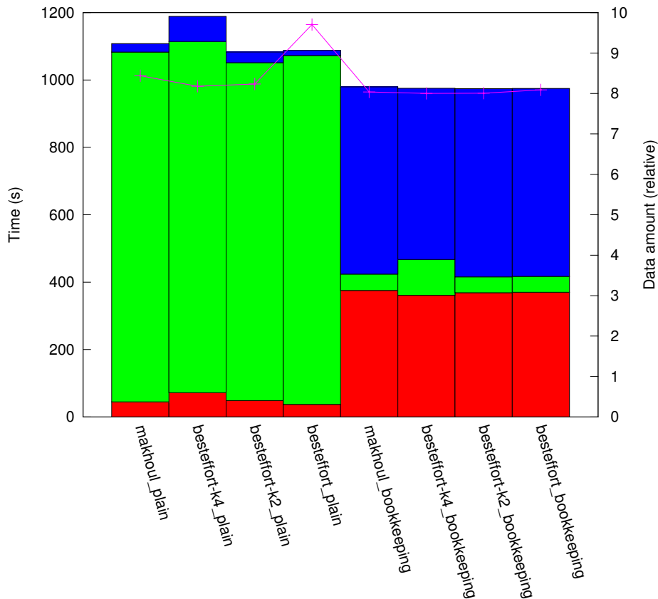
results_R1_1:1/plat_grid256/topo_torus
