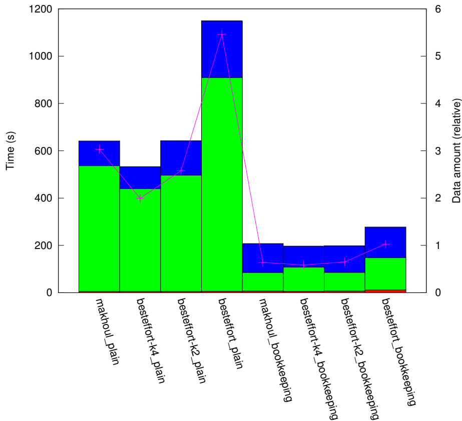
results_RN_1:10/plat_grid256/topo_torus
