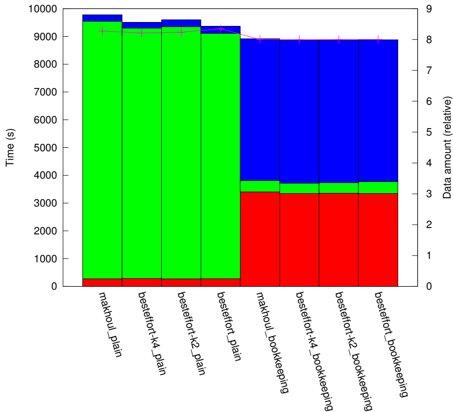
results_l1_1:10/plat_grid256/topo_torus
