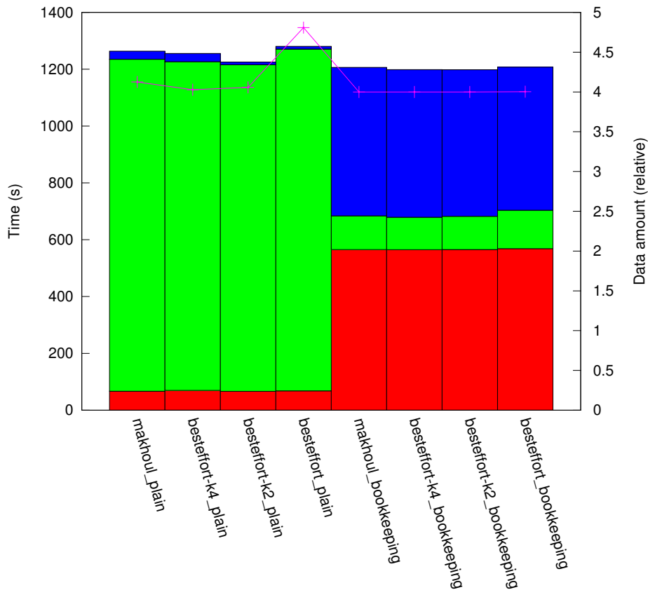
results_I1_1:10/plat_cluster64/topo_torus
