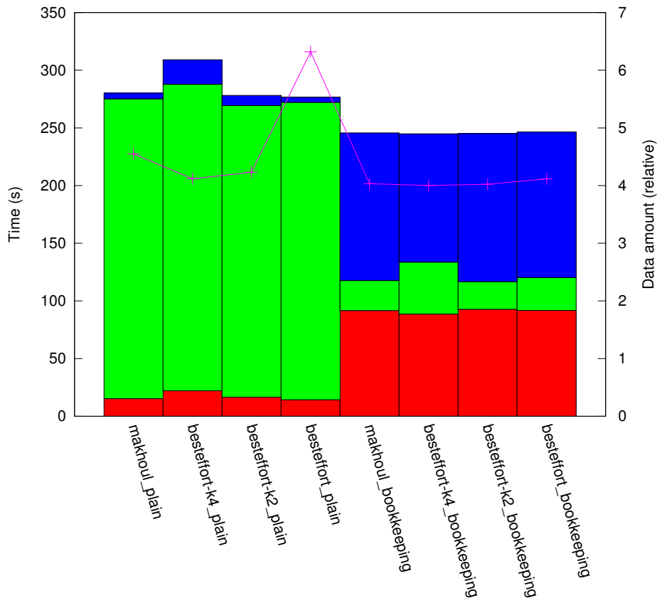
results_R1_1:1/plat_grid64/topo_torus
