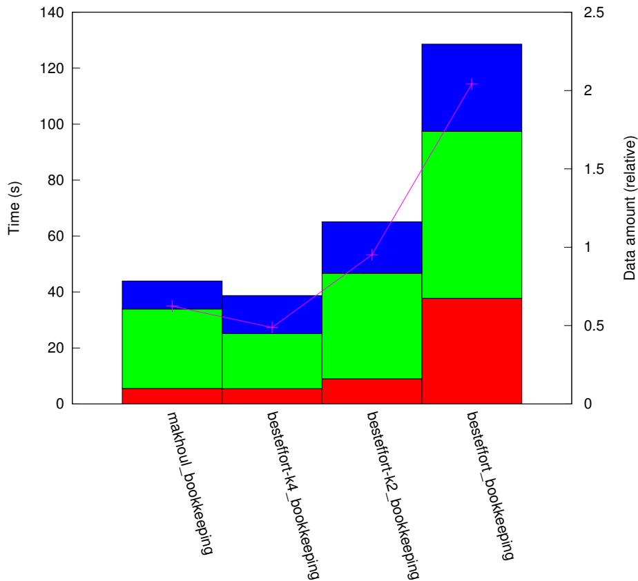
results_RN_1:1/plat_grid1024/topo_hcube
