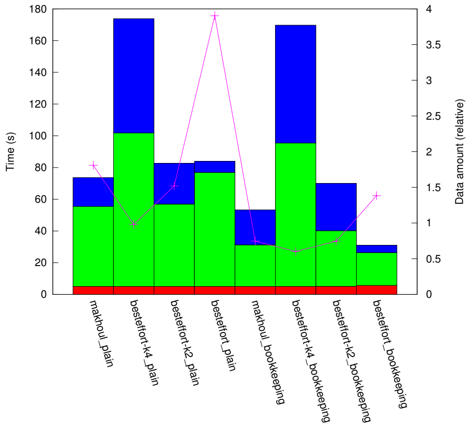
results_RN_1:1/plat_cluster256/topo_torus
