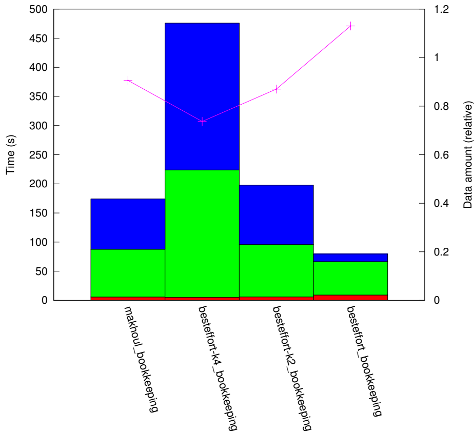
results_RN_1:1/plat_cluster1024/topo_torus
