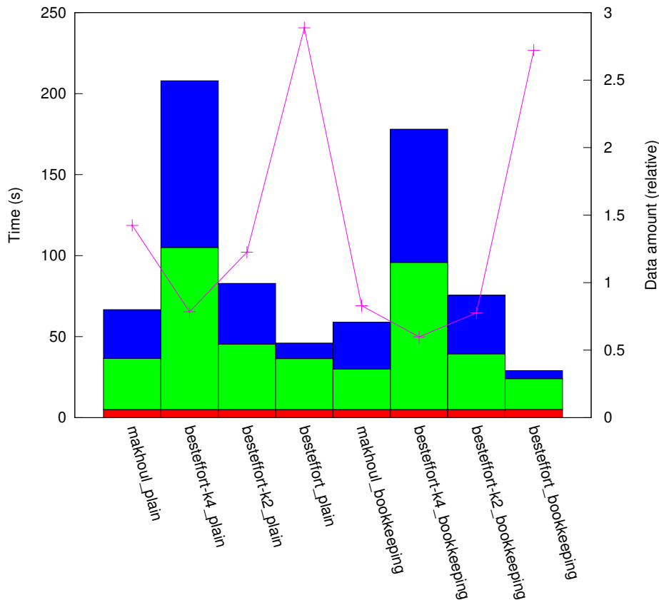
results_IN_10:1/plat_cluster256/topo_torus
