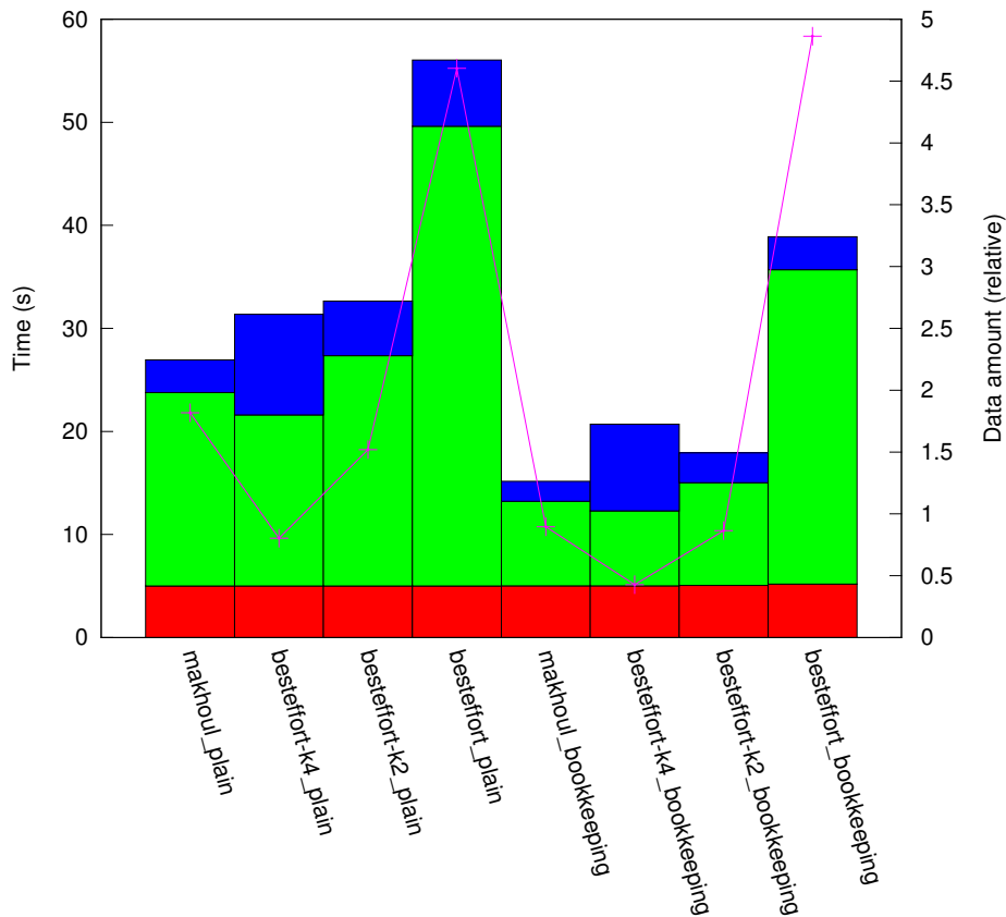
results_RN_10:1/plat_grid64/topo_hcube
