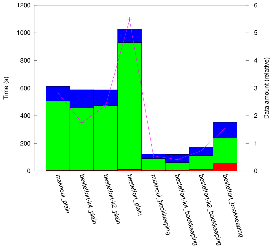
results_IN_1:10/plat_cluster256/topo_hcube
