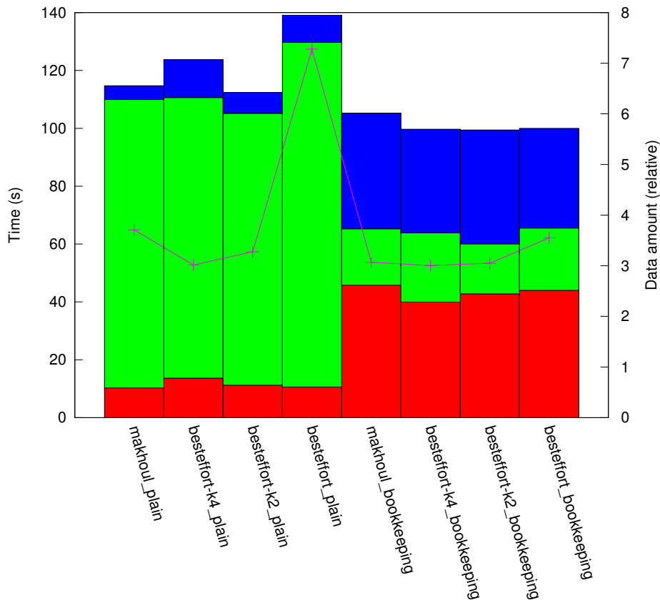
results_R1_1:1/plat_cluster64/topo_hcube
