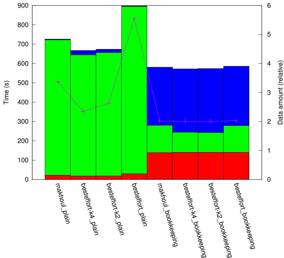
results_R1_1:10/plat_grid16/topo_torus
