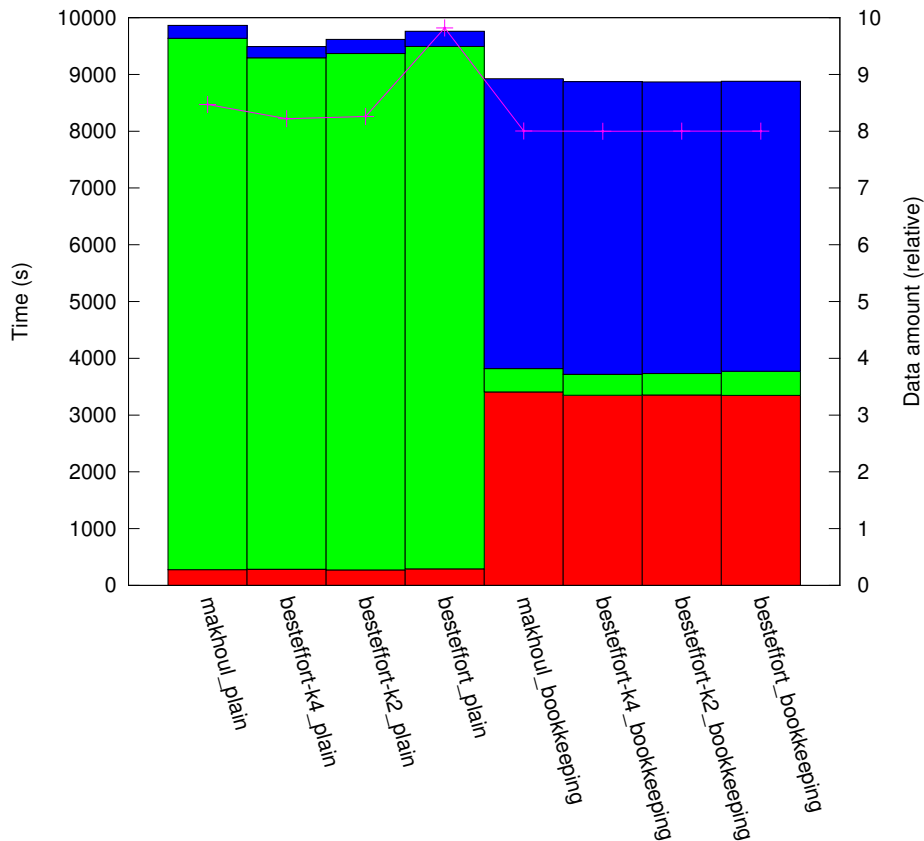
results_R1_1:10/plat_grid256/topo_torus
