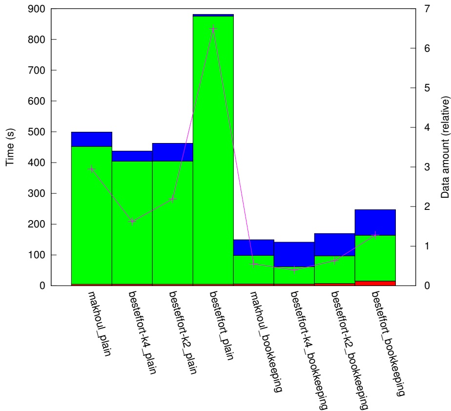
results_RN_1:10/plat_grid64/topo_hcube
