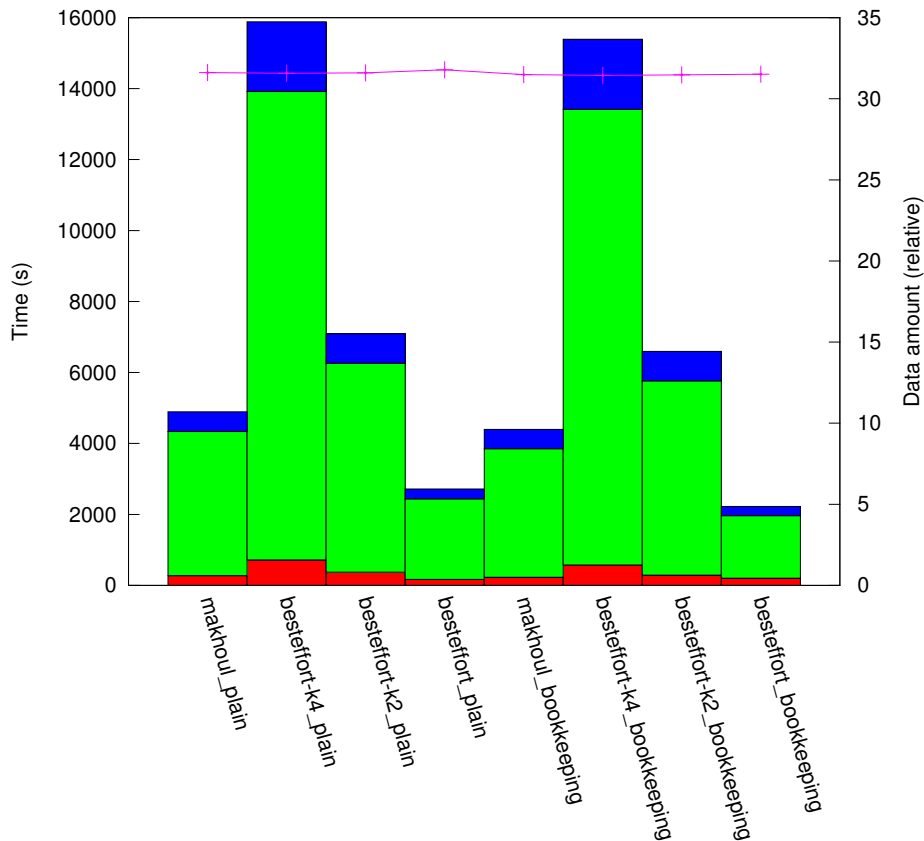
results_R1_1:1/plat_cluster64/topo_line
