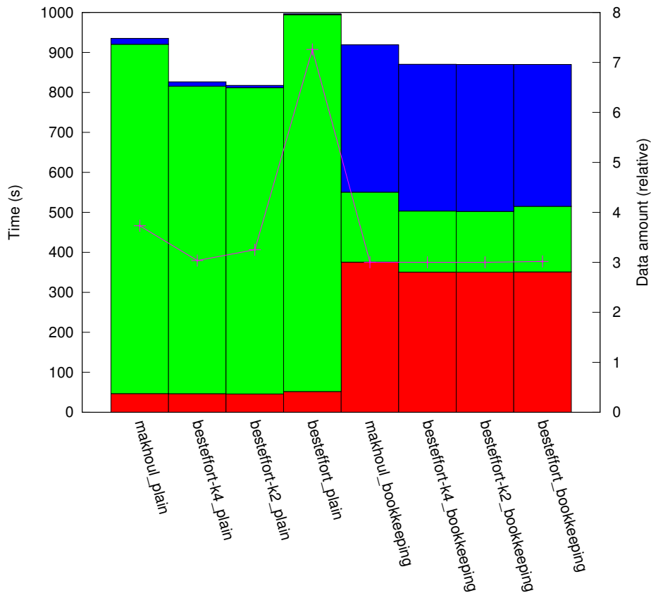
results_R1_1:10/plat_cluster64/topo_hcube
