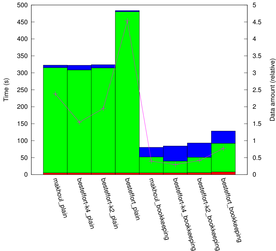
results_RN_1:10/plat_cluster16/topo_torus
