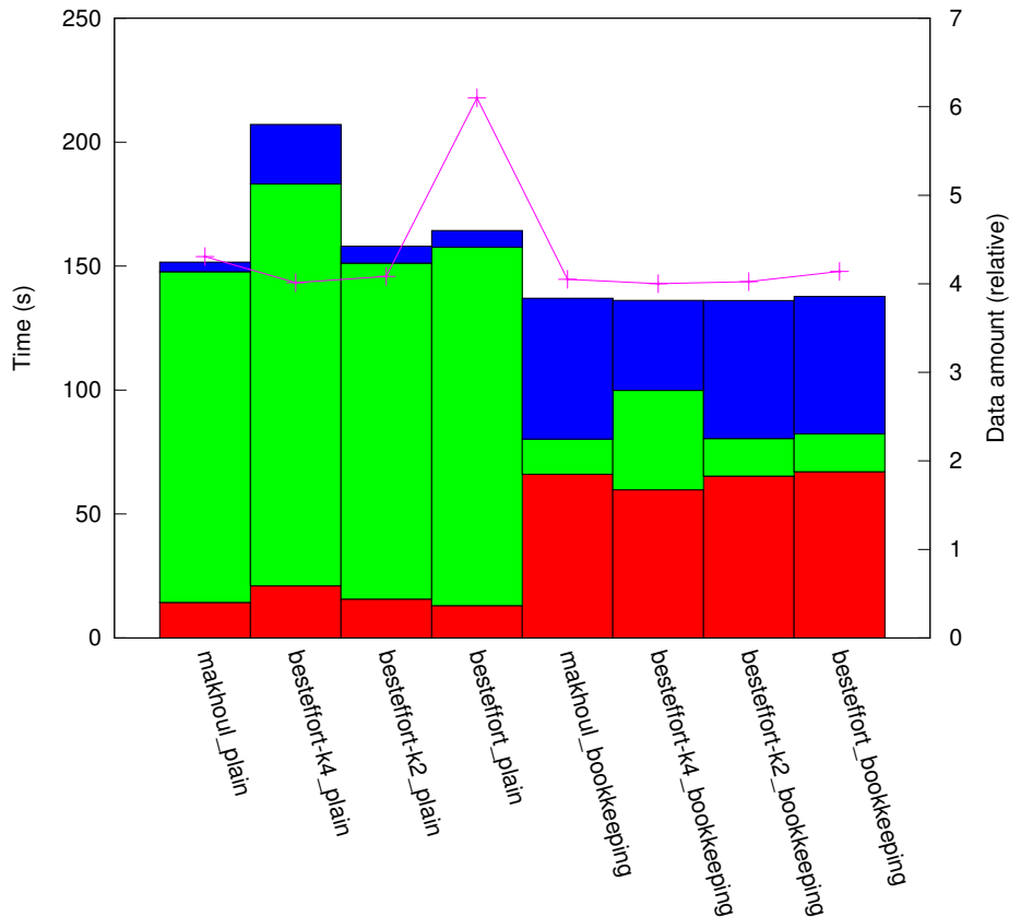
results_R1_1:1/plat_cluster64/topo_torus
