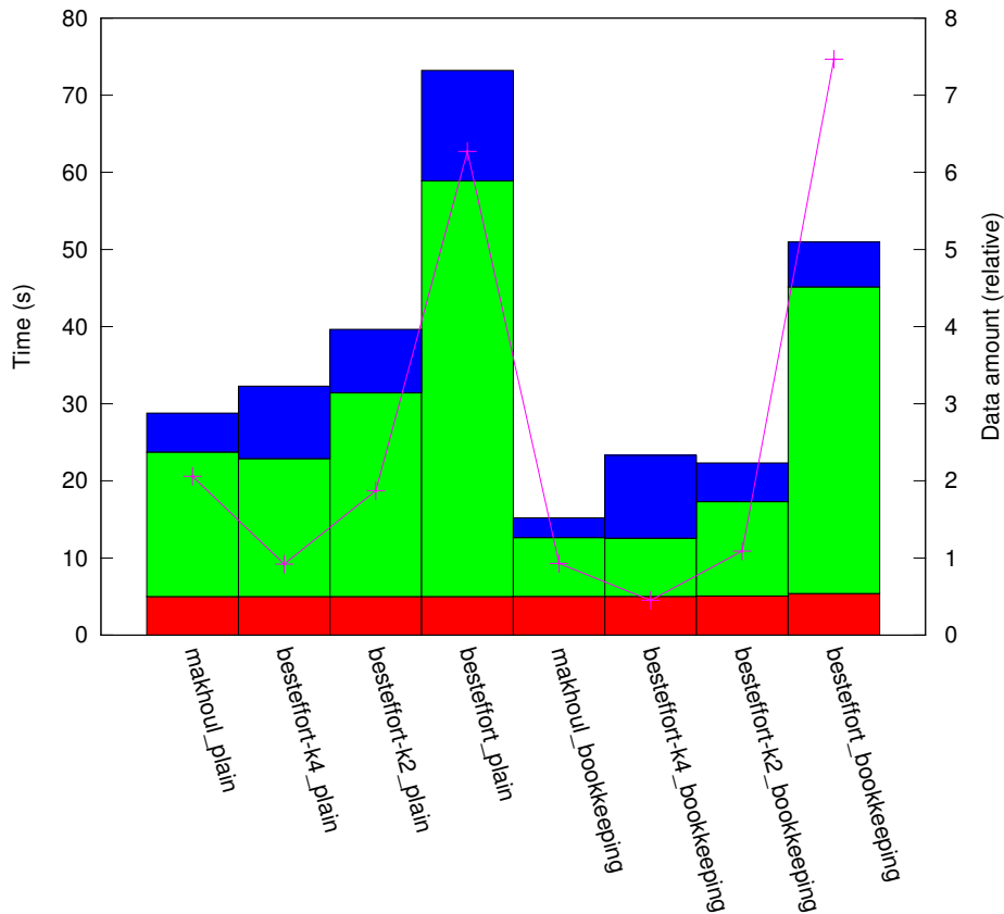
results_IN_10:1/plat_cluster256/topo_hcube
