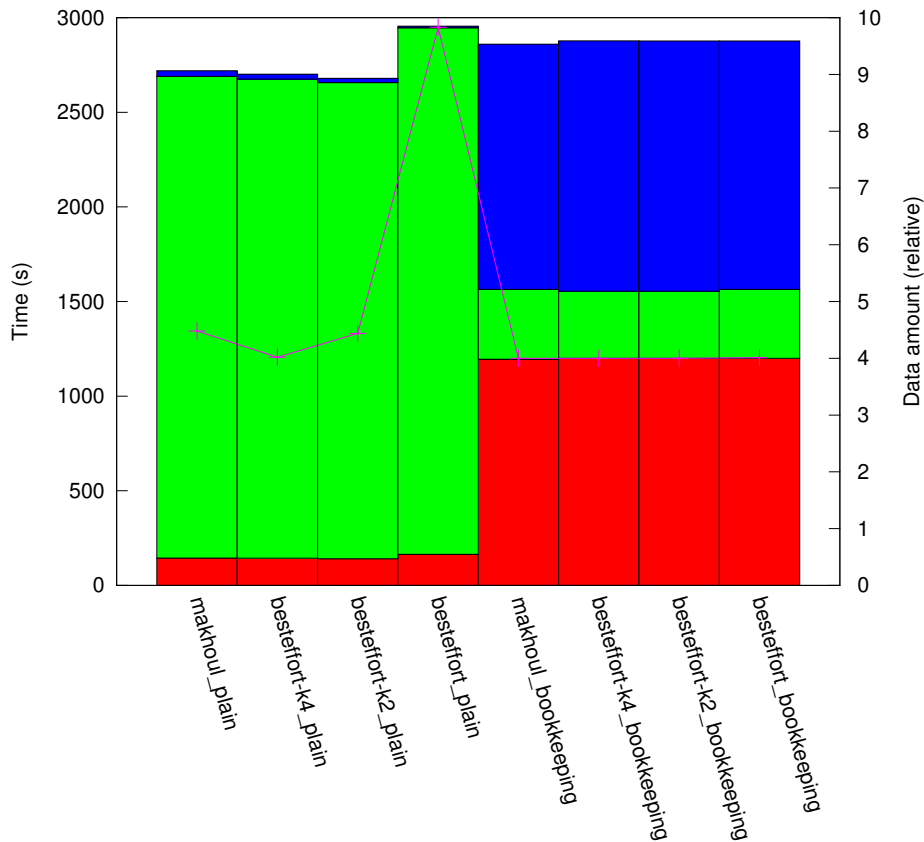
results_R1_1:10/plat_cluster256/topo_hcube
