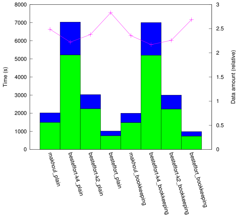
results_RN_10:1/plat_cluster64/topo_line
