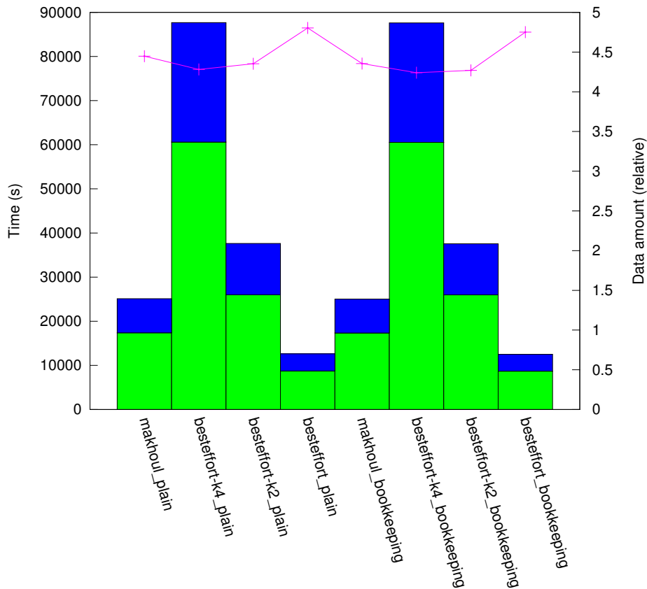
results_RN_10:1/plat_grid256/topo_line
