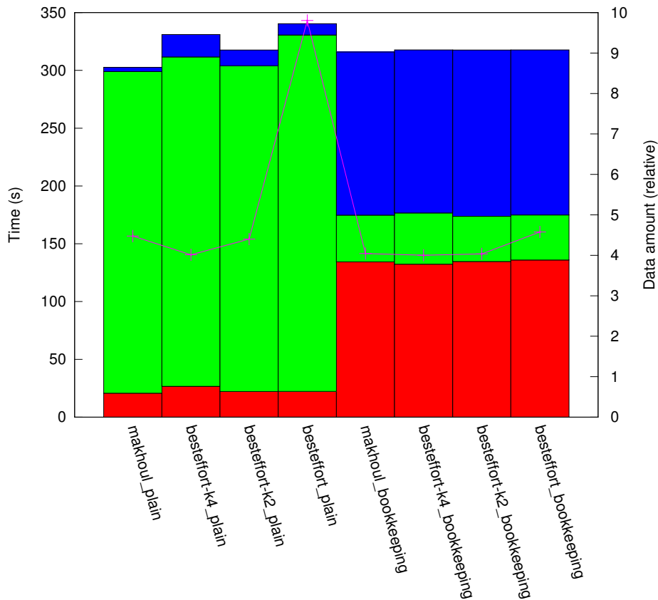
results_R1_1:1/plat_cluster256/topo_hcube
