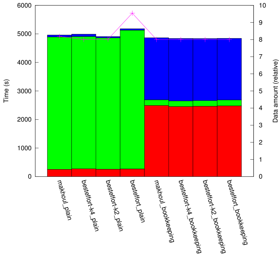
results_R1_1:10/plat_cluster256/topo_torus
