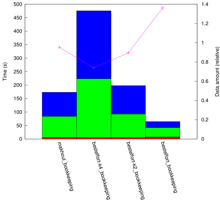
results_RN_1:1/plat_grid1024/topo_torus
