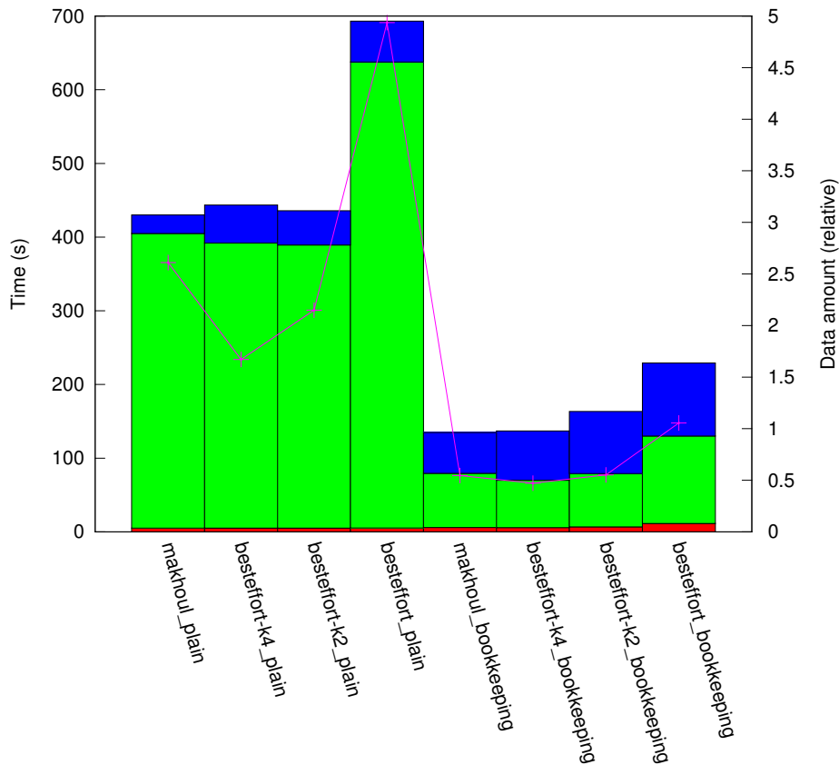
results_RN_1:10/plat_grid64/topo_torus
