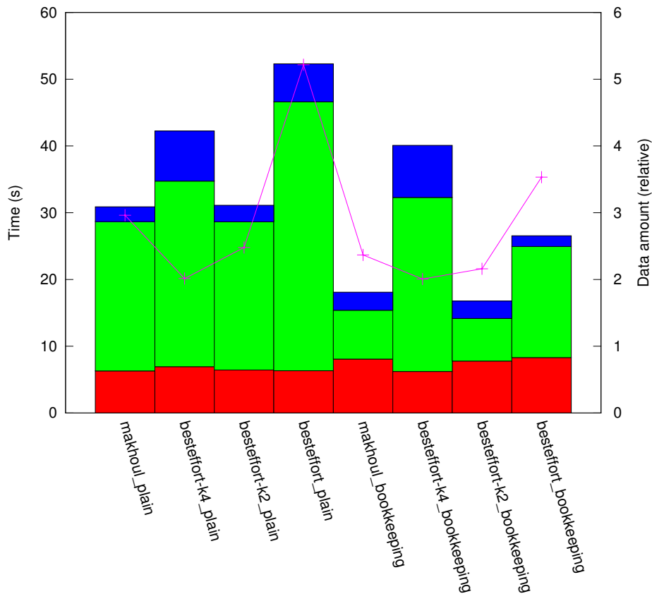
results_R1_10:1/plat_grid16/topo_torus
