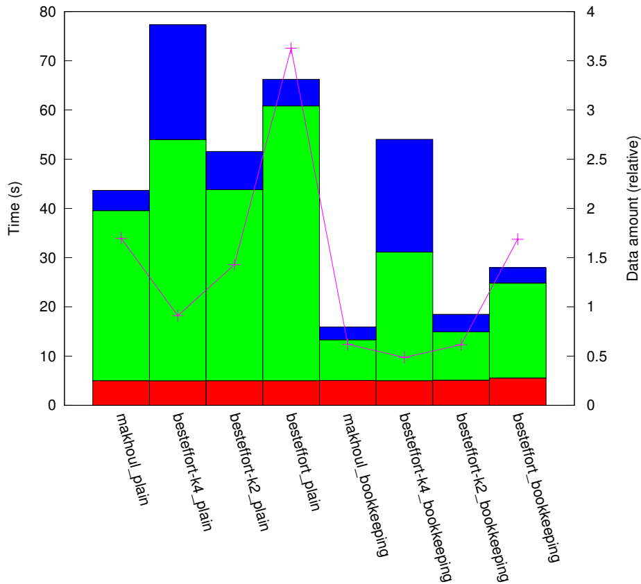
results_RN_1:1/plat_cluster64/topo_torus
