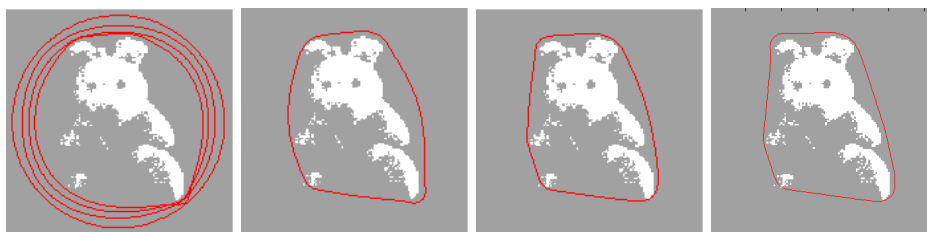
(a) Les états initial et (b) L'état du contour (c) L'état du contour (d) L'état du contour suivant chacune des après la septième ité- après la dixième ité- après la centième itérations trois premières itéra- ration ration itération. C'est le contour final.
