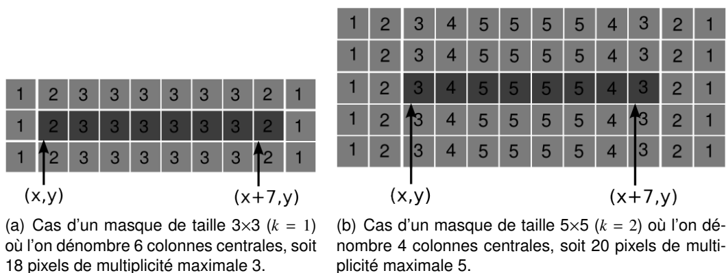
FIGURE 9.1 – Multiplicité des implications des pixels de la zone d'intérêt d'un thread dans les calculs de convolution. Le nombre de calculs dans lequel est impliqué un pixel est inscrit en son centre. Le premier pixel du paquet, ou pixel de base, est repéré par ses coordonnées (x, y) ; le dernier à pour coordonnées (x + 7, y)
