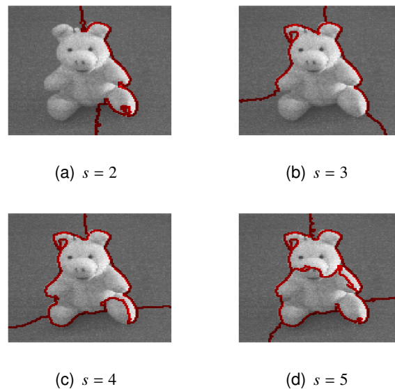
FIGURE 2.2 – Segmentation d’une image en niveaux de gris de 128 \times 128 pixels par simplification de graphe de type Normalized cut pour un nombre s de segments variant de 2 à 5.
