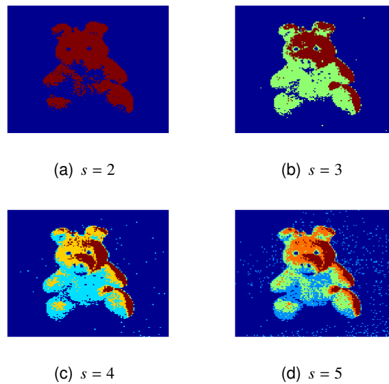
FIGURE 2.3 – Segmentation d’une image en niveaux de gris de 128 \times 128 pixels par algorithme k-means pour un nombre s de segments variant de 2 à 5. Chaque couleur est associée à un segment. Les couleurs sont choisies pour une meilleure visualisation des différents segments.
