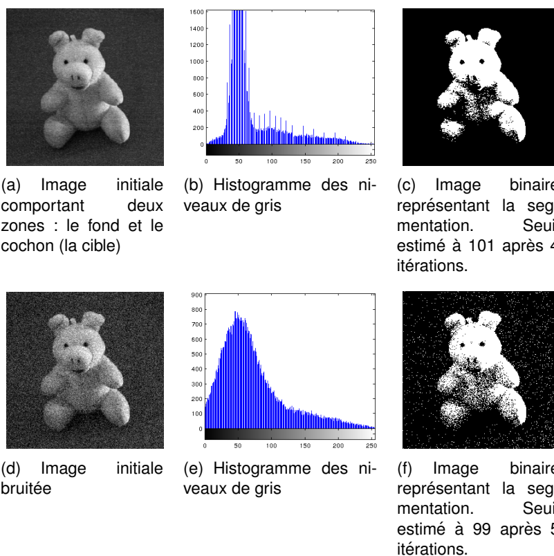
FIGURE 2.1 – Segmentation d’une image en niveaux de gris de 128 \times 128 pixels par analyse simple d’histogramme. Colonne de gauche : image d’entrée. Colonne centrale : histogramme des niveaux de gris. Colonne de droite : résultat de la segmentation.
