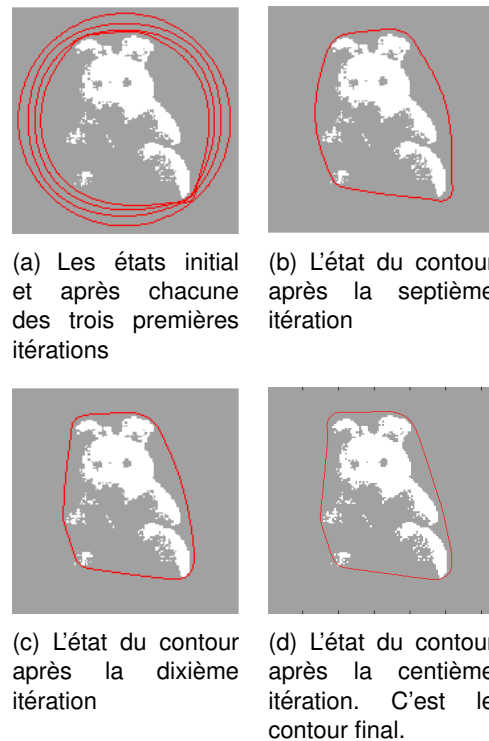
FIGURE 2.5 – Segmentation d’une image en niveaux de gris de 128 \times 128 pixels par algorithme dit du snake , dans sa version originale. Les paramètres d’élasticité, de viscosité, de raideur et d’attraction ont été fixés respectivement aux valeurs 5, 0, 0.1 et 5.
