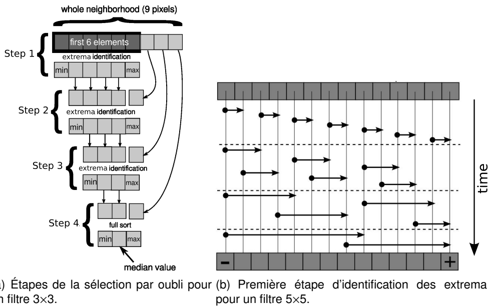
FIGURE 6.1 – Application de la sélection de médiane par oubli. a) à une fenêtre de 3 × 3 pixels. b) Maximisation de l’ILP pour l’identification des extrema.
