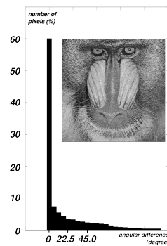
FIGURE 5.6 – Histogramme des écarts angulaires entre la direction primaire de l' isoline optimale et celle de l' isoline sélectionnée, pour l'image du singe (Mandrill). Pour la très grande majorité des pixels, le mode de sélection de l' isoline ne génère pas d'erreur sur la direction du premier segment.
