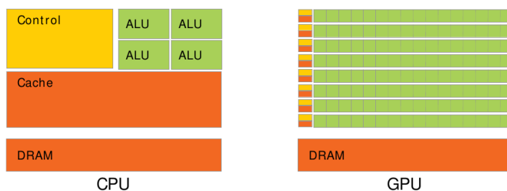
FIGURE 2.1 – Comparaison des structures d'un cœur de GPU et d'un cœur de CPU (d'après [64]). ALU = Arithmetical & Logical Unit.
