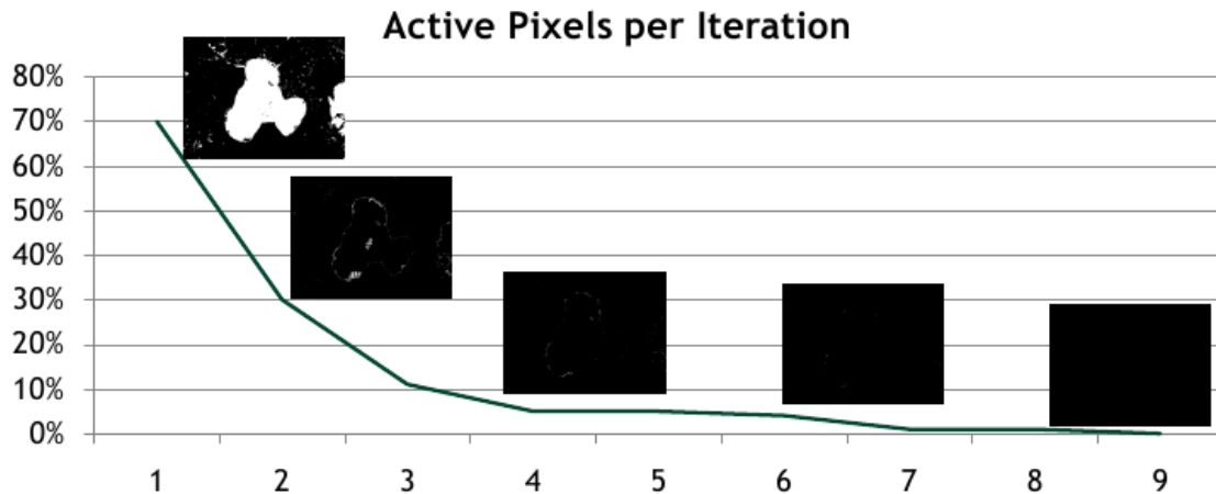
FIGURE 3.15 – Évolution du nombre de pixels actifs pour les itérations successives de l'implémentation de l'algorithme push-relabel de [84]. Les petites images montrent la localisation des pixels actifs après chaque itération, en blanc.
