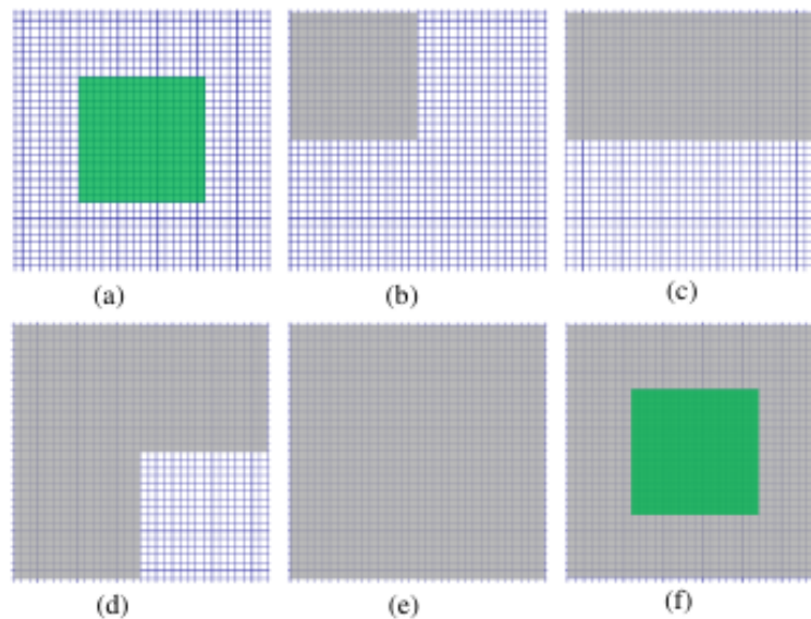
FIGURE 3.9 – Illustration du pré-chargement en mémoire partagée mis en œuvre dans [102] pour l'implémentation, entre autres, du filtre bilatéral. a) en vert le bloc de threads associé aux pixels centraux. b-e) les blocs de pixels successivement pré-chargés en mémoire partagée. f) la configuration finale de la ROI en mémoire partagée.
