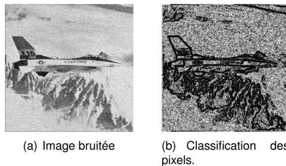
FIGURE 5.12 – Classification des pixels d'une image bruitée, pour une valeur de seuil T_2 = 2 du détecteur. b) Les pixels en noir sont ceux à qui le PI-PD sera appliqué. Les pixels en blancs se verront appliquer une moyenne sur tout ou partie du voisinage.
