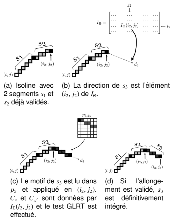
FIGURE 5.8 – Exemple d'application du procédé d'allongement à une isoline comprenant initialement 2 segments. la longueur des segments est d = 5 . Le procédé se répète jusqu'à ce que le test GLRT échoue.
