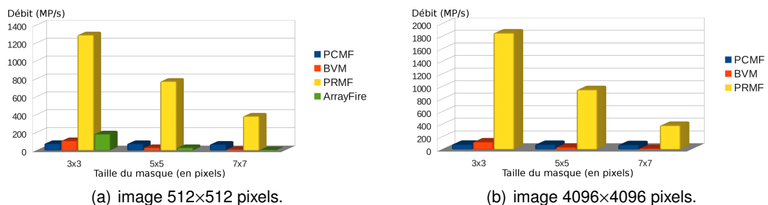
FIGURE 6.3 – Comparaison des débits (MP/s) atteints par notre implémentation notée PRMF, avec les principales solutions de référence. De gauche à droite : PCMF, BVM, PRMF, ArrayFire (impossible en 4096x4096)
