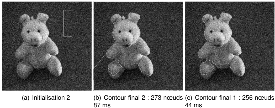
FIGURE 4.3 – Influence du contour initial sur la segmentation. Le contour final 1 est celui de la figure 4.2.
