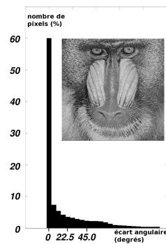
FIGURE 5.6 – Histogramme des écarts angulaires entre la direction primaire de l’isoline optimale et celle de l’isoline sélectionnée, pour l’image du singe (Mandrill). Pour la très grande majorité des pixels, le mode de sélection de l’isoline ne génère pas d’erreur sur la direction du premier segment.
