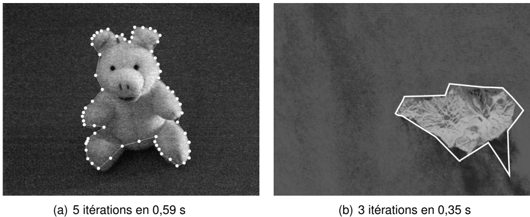
FIGURE 4.11 – Segmentations de grandes images, avec le contour initial transposé de celui de la figure 4.2. a) image du cochon en 100 MP. b) image satellite de l’île de Montserrat en 150 MP.
