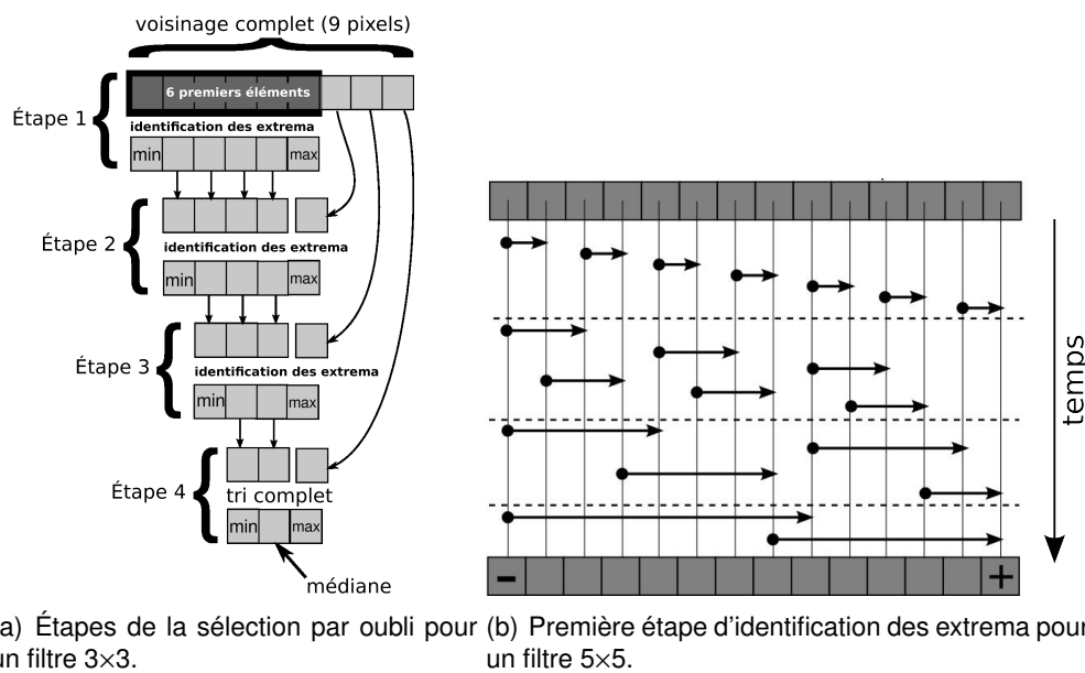
FIGURE 6.1 – Application de la sélection de médiane par oubli. a) à une fenêtre de 3 \times 3 pixels. b) Maximisation de l’ILP (Instruction Level Parallelism) pour l’identification des extrema.
