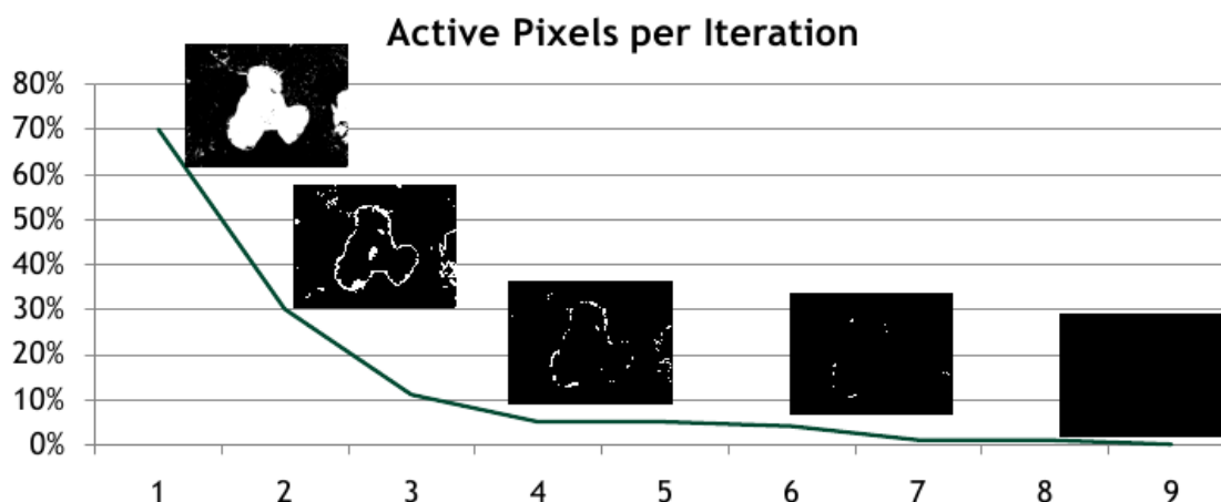
FIGURE 5.6 – Évolution du nombre de pixels actifs pour les itérations successives de l'implémentation de l'algorithme push-relabel de [94]. Les petites images montrent la localisation des pixels actifs après chaque itération, en blanc.
