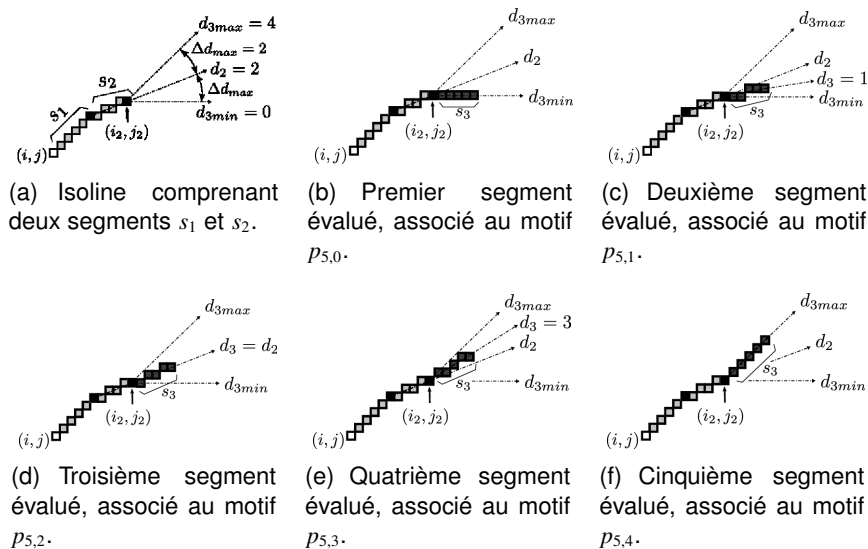
FIGURE 7.5 – Processus de sélection lors de l'allongement d'une isoline comportant initialement deux segments s_1 et s_2 . Dans cet exemple a = 5 et \Delta d_{max} = 2 . Chaque segment évalué est soumis au test GLRT. Si au moins un des segments présente un test GLRT positif, alors l'allongement est réalisé avec le segment qui forme l'isoline la plus vraisemblable.
