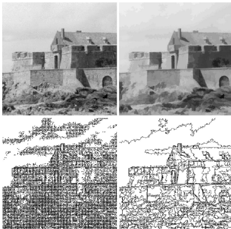
FIGURE 7.1 – Exemple d'exploitation des lignes de niveaux. En haut : l'image originale et sa représentation à l'échelle \times 150 . En bas : les lignes de niveaux de l'image originale et celles utilisées pour la mise à l'échelle. Toutes les lignes de niveaux de l'image de droite existent à l'identique dans l'ensemble original. Illustration tirée de [16].
