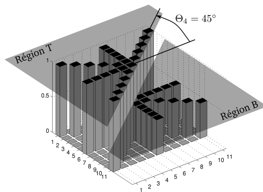
FIGURE 7.12 – Motif de détection des zones à faible pente, pour le cas \Theta = \Theta_4 = 45^\circ . L'élévation des pixels permet juste de les distinguer selon 3 classes : l'élévation 1 est associée aux pixels de la région T , l'élévation 0.5 est associée à ceux de la région B et l'élévation 0 désigne les pixels n'intervenant pas dans la détection.
