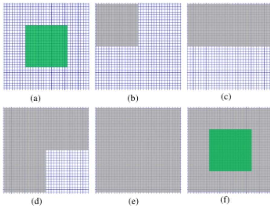
FIGURE 4.9 – Illustration du pré-chargement en mémoire partagée mis en œuvre dans [113] pour l’implémentation, entre autres, du filtre bilatéral. a) en vert le bloc de threads associé aux pixels centraux. b-e) les blocs de pixels successivement pré-chargés en mémoire partagée. f) la configuration finale de la ROI en mémoire partagée.
