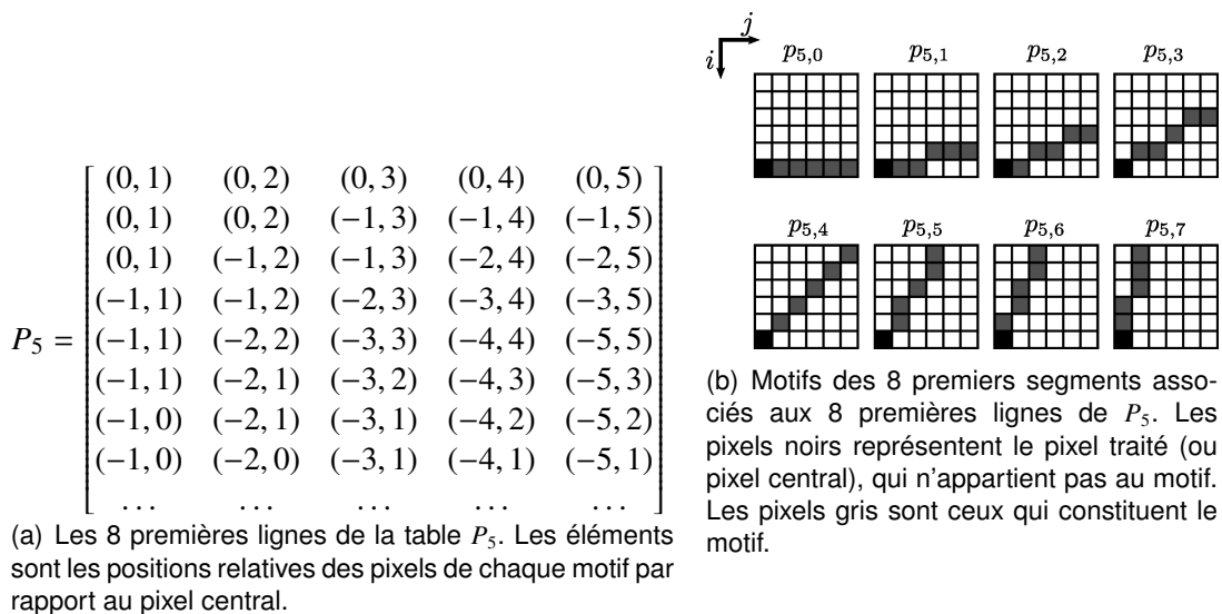
FIGURE 7.2 – Détail des motifs et de leur représentation interne, pour la taille a = 5 .
