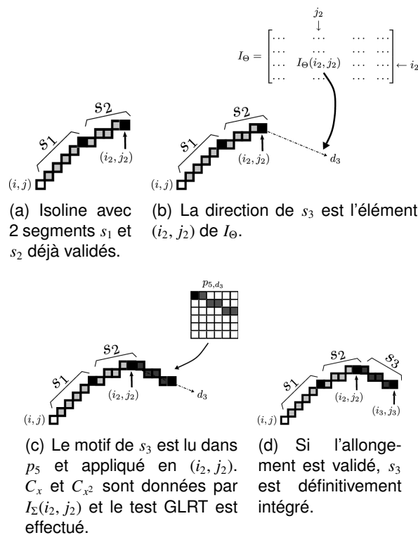
FIGURE 7.9 – Exemple d'application du procédé d'allongement à une isoline comprenant initialement 2 segments. la longueur des segments est a = 5 . Le procédé se répète jusqu'à ce que le test GLRT échoue.
