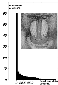
FIGURE 7.7 – Histogramme des écarts angulaires entre la direction primaire de l’isoline optimale et celle du segment sélectionné par PI-LD avec q = 1 (sans allongement), pour l’image du singe (Mandrill). Pour la très grande majorité des pixels, l’écart est nul.
