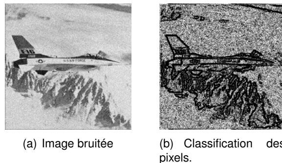
FIGURE 7.13 – Classification des pixels d'une image bruitée, pour une valeur de seuil T_2 = 2 du détecteur. (b) Les pixels en noir sont ceux à qui le PI-PD sera appliqué. Les pixels gris se verront appliquer une moyenne sur tout ou partie du voisinage.
