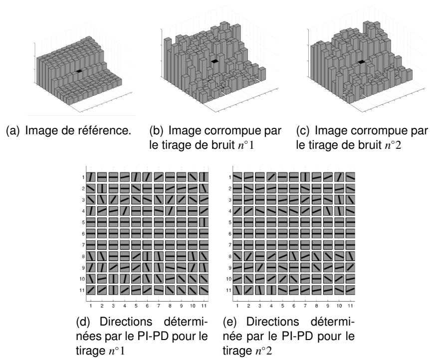
FIGURE 7.11 – Comportement du modèle PI-PD dans les zones de faible et à forte pente. On constate un manque de robustesse dans les zones à faible pente : les directions ne sont pas reproduites d'un tirage à l'autre, contrairement à celles de la zone de transition.
