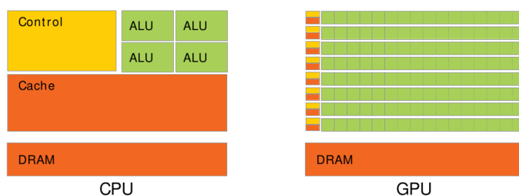
FIGURE 2.1 – Comparaison des structures d'un cœur de GPU et d'un cœur de CPU (d'après [69]). ALU = Arithmetical & Logical Unit.
