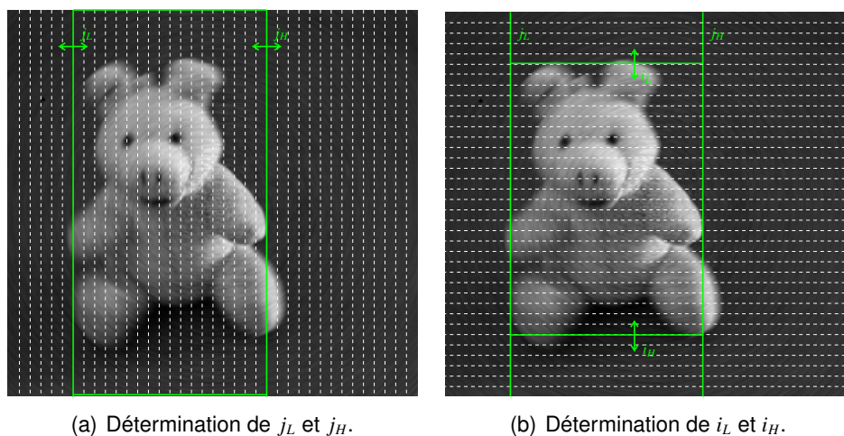
FIGURE 6.12 – Détermination intelligente du contour initial en deux phases successives. (a) La première étape repose sur un échantillonnage horizontal. (b) La seconde étape repose sur un échantillonnage vertical.
