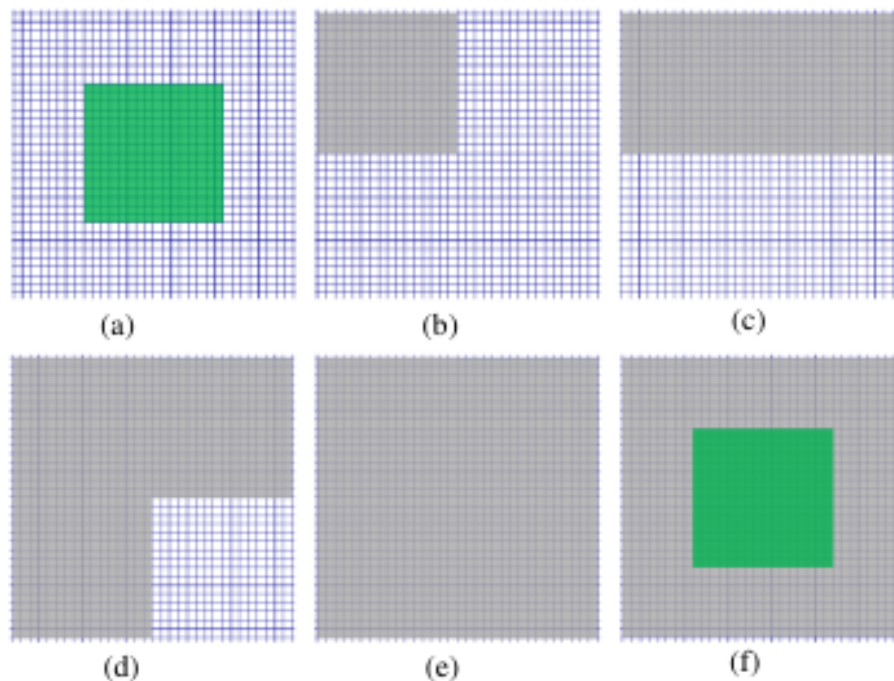
FIGURE 4.9 – Illustration du pré-chargement en mémoire partagée mis en œuvre dans [111] pour l’implémentation, entre autres, du filtre bilatéral. a) en vert le bloc de threads associé aux pixels centraux. b-e) les blocs de pixels successivement pré-chargés en mémoire partagée. f) la configuration finale de la ROI en mémoire partagée.
